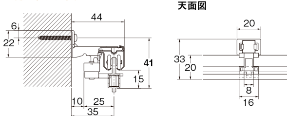
カバートップIIセット平面図
