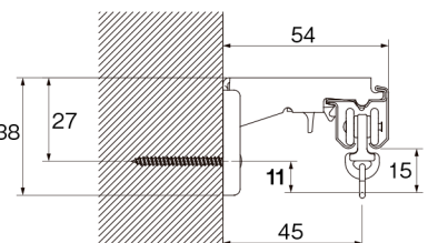
LTエキストラシングルブラケット付 (ブラケット幅=35mm)
