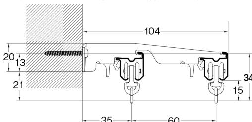
NTダブルブラケット付 (ブラケット幅=44mm)
