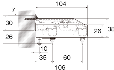
カバートップIIセット側面図
