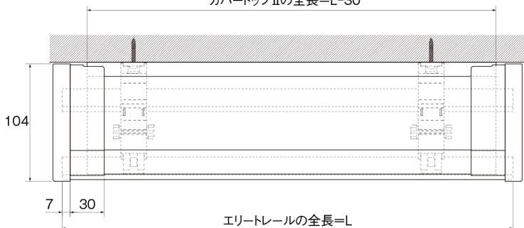
カバートップIIセット平面図
