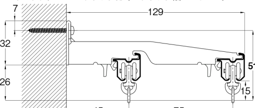
エキストラダブルブラケット付 (ブラケット幅=18mm)
