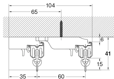
天井付ダブルブラケットII付 (ブラケット幅=21mm)
